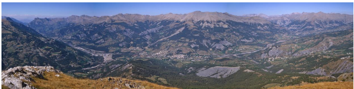
Vue d'ensemble de la vallée de Barcelonnette, depuis le sud. Il s'agit d'une "fenêtre" structurale, avec au fond de la vallée les sédiments du domaine dauphinois (principalement les Terres Noires du Jurassique moyen), recouverts par les nappes de l'Embrunais-Ubaye, essentiellement constituées de Flysch à Helminthoïdes qui forme les crêtes dépourvues de végétation à l'arrière-plan.
