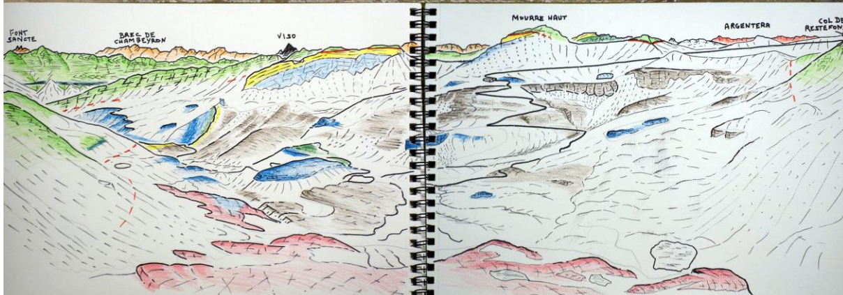
Mercredi 24/09: environs du col de Restefond. Panorama et dessin depuis le Pas de Touréris, avec le Nummulitique (grès d'Annot, gris) recouvert par des "écaïlles" de séries subbriançonnaises (bleu foncé), briançonnaises (rose) et provençales (bleu clair/jaune), puis par les nappes de Flysch à Helminthoïdes (vert).
