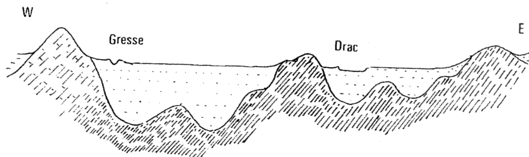
Coupe transversale de la plaine du Drac, au Sud de Grenoble.
